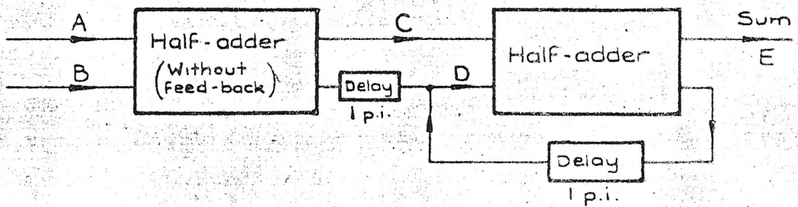
Fig. 4(b) ADDER
