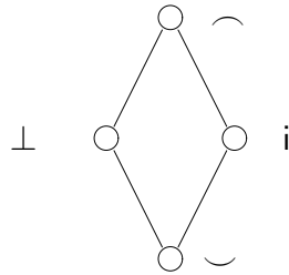
Fig. 2. The poset 4
